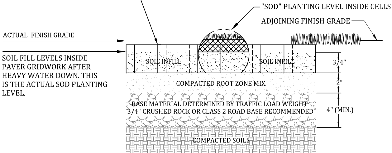
EZ ROLL GRASS ROAD PAVER
